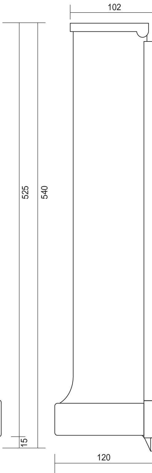
側面図
